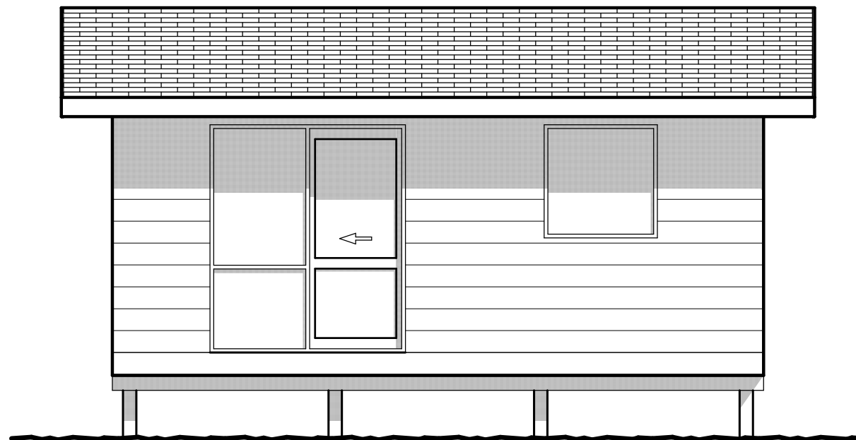
ELEVATION 3
