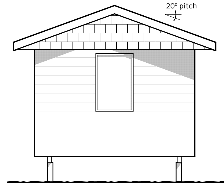
ELEVATION 4
