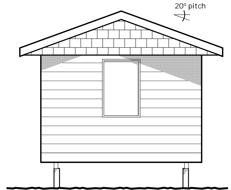
ELEVATION 2
